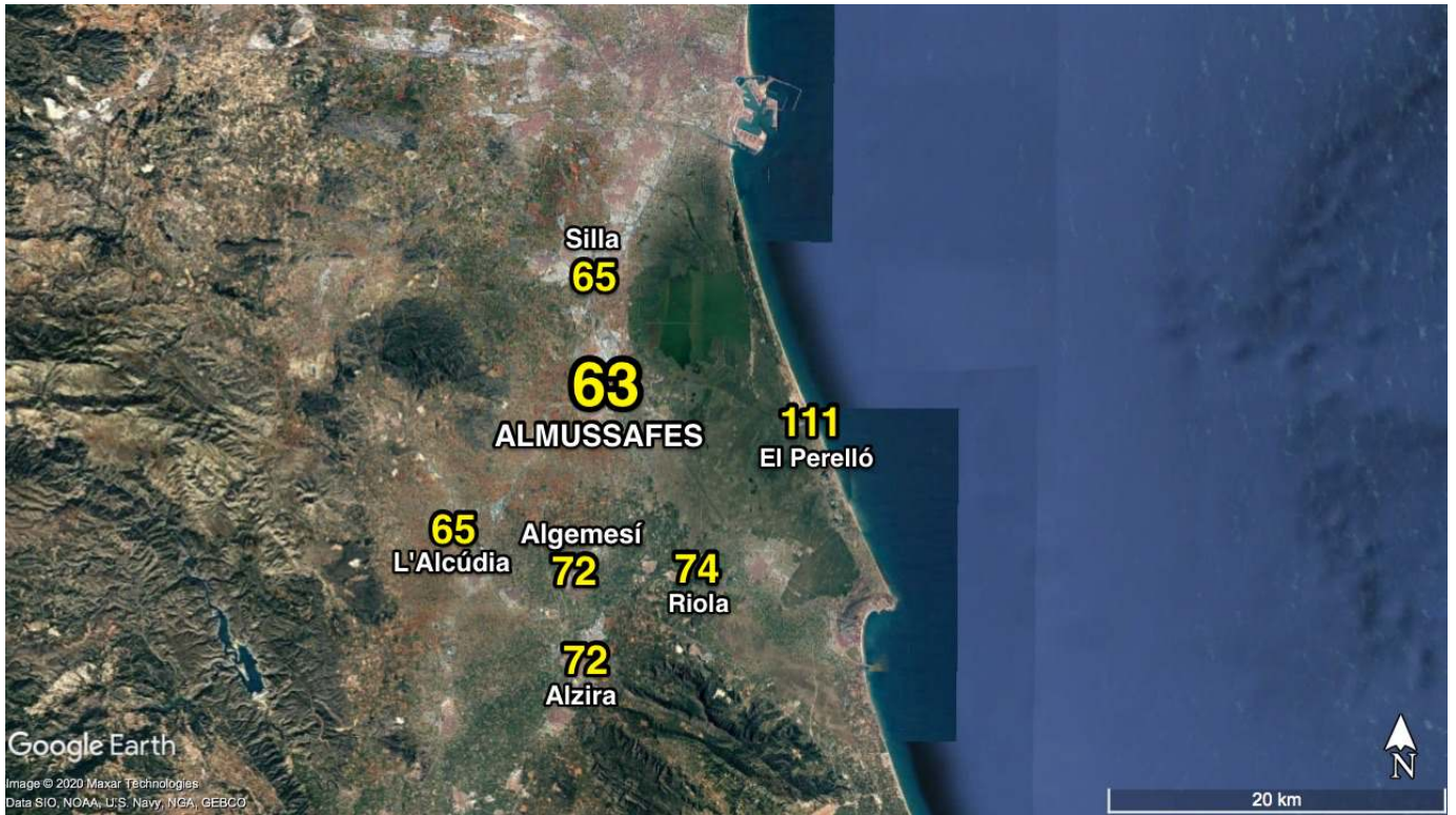
Ráfagas máximas de viento registradas en ALMUSSAFES y alrededores entre el 19 y el 22/01/20 (en km/h)
