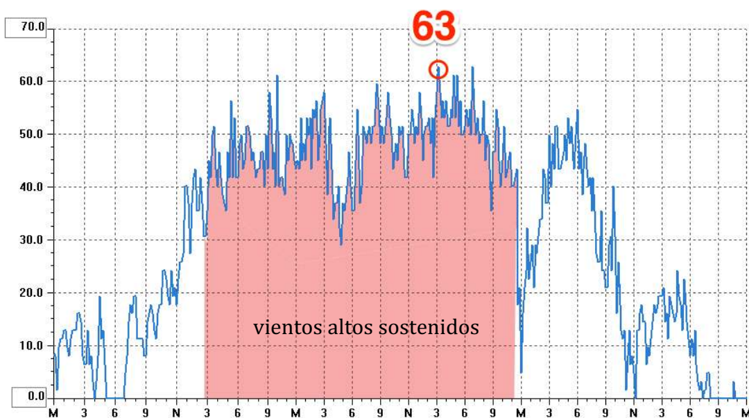
Ráfagas de viento registradas por la estación municipal de ALMUSSAFES entre el 19 y el 21/01/20 (en km/h)
