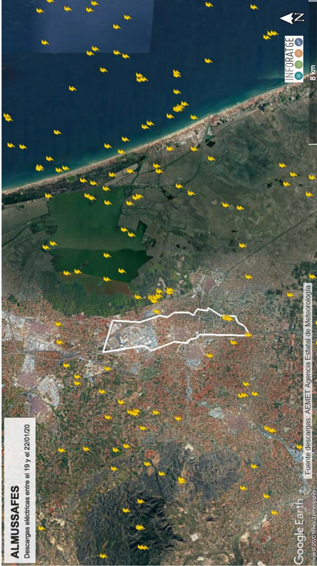
Geolocalización de las descargas eléctricas ~ nube-tierra registradas en el término municipal de ALMUÑAFES y alrededores entre el 19 y el 22/01/20 Fuente descargas: AEMET Agencia Estatal de Meteorología
